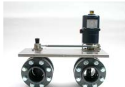
Mengklep VDL+OMa
